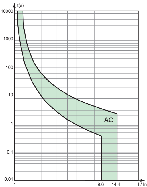
D曲线
