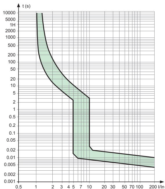
C曲线
